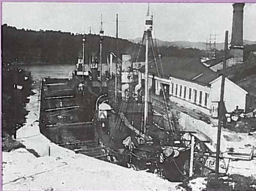
I steindokken på Bredalsholmen utenfor Kristiansand fikk i sin tid mang en skute en overhaling før det bar til havs igjen. Dokken, som er bygd i 1873-76 og tilhører Kristiansands Mekaniske Verksted, blir nå satt i stand og bevart som et teknisk kulturminne. (Foto: Smestad Foto)
